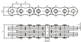
鏈板組合 Plate lacing
